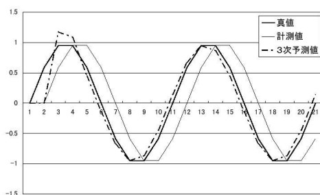
図 D.3 予測フィルタの動作シミュレーション (3 次予測の場合)
