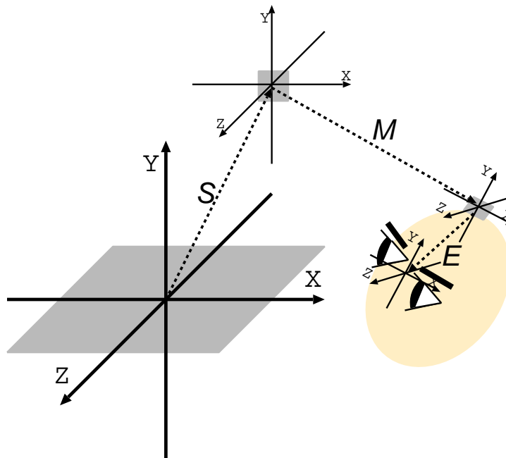
図 B.1 3次元座標変換パラメータ
