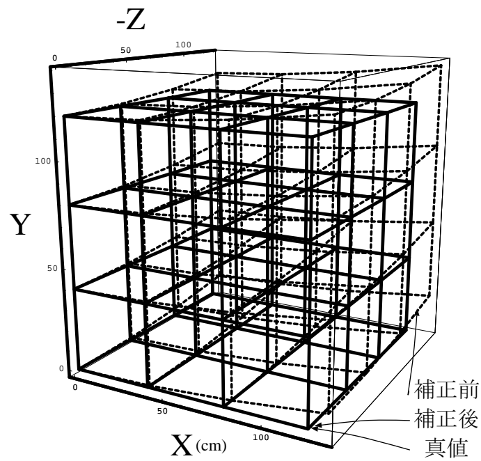
図 C.1 磁場補正のシミュレーション（誤差の大きい場合）
