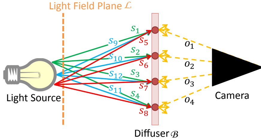
図 6 提案手法の概念図.
