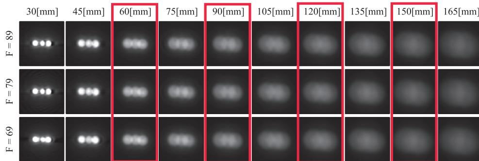
図 24 実球面調和関数の次数を F = 69, 79, 89 とした場合における提案手法 (I) によって推定した放射輝度分布を用いてリライティングした画像. 図中赤枠で囲まれた領域は放射輝度分布の推定に用いた撮影画像に対応している. なお図中の画像は拡大表示されている.
