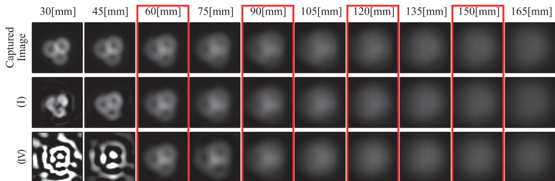
図 29 LED が三角形状態に配列された光源を用いた場合における撮影画像 (真値) と各手法によって推定された放射輝度分布を用いてリライティングした画像. (I) L1 ノルム正則化と物理制約を用いた手法, (IV) 制約条件を用いない手法. 実球面調和関数の次元を 34 とし, 空間方向の解像度を 35 として放射輝度分布を推定. 図中赤枠で囲まれた領域は放射輝度分布の推定に用いた撮影画像に対応している. なお図中の画像は拡大表示されている.
