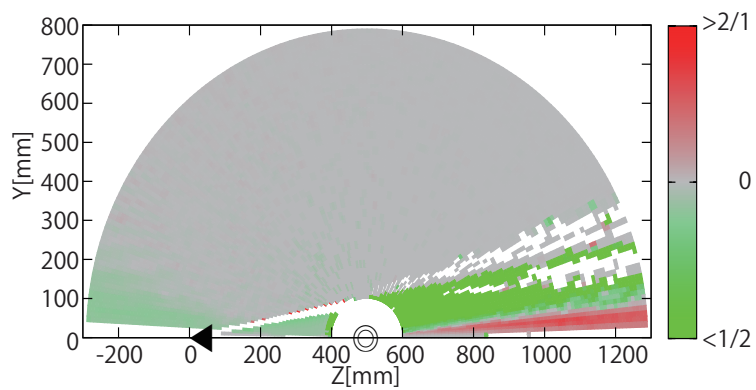
(a) 中空透明球体. 中点法 ( \sigma = 1.0 , 厚さ 0mm )
