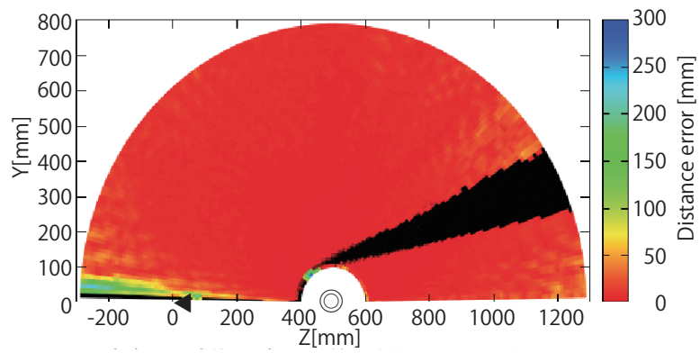
(a) 中空透明球体. 再投影誤差最小化 ( \sigma = 0 , 厚さ 0\text{mm} )
