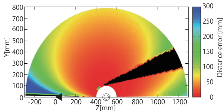
(b) 中空透明球体. 再投影誤差最小化 ( \sigma = 1.0 , 厚さ 0\text{mm} )
