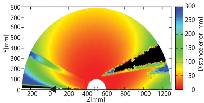
(b) 中空透明球体. 再投影誤差最小化 ( \sigma = 1.0 , 厚さ 2\text{mm} , 屈折率 1.5) 球の厚みを考慮して光源位置を推定
