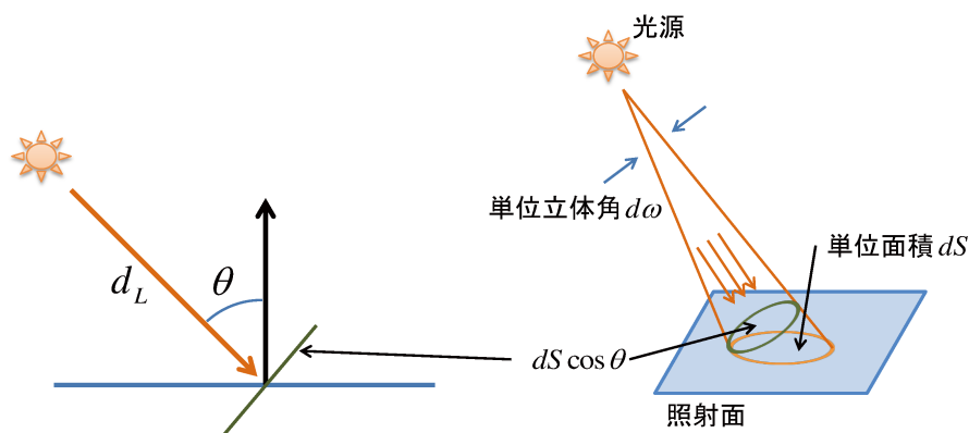
図 49 光源と物体表面
