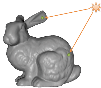
図 2 近接光源の場合における物体表面に入射する光の角度
