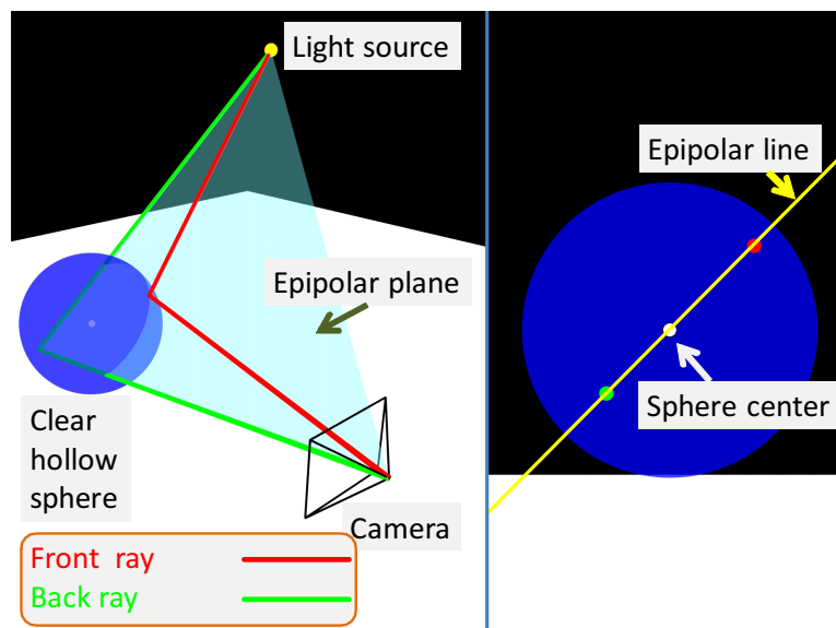
図 31 中空透明球体を用いたエピポーラ幾何. 左: 外観図 右: 観測画像.
