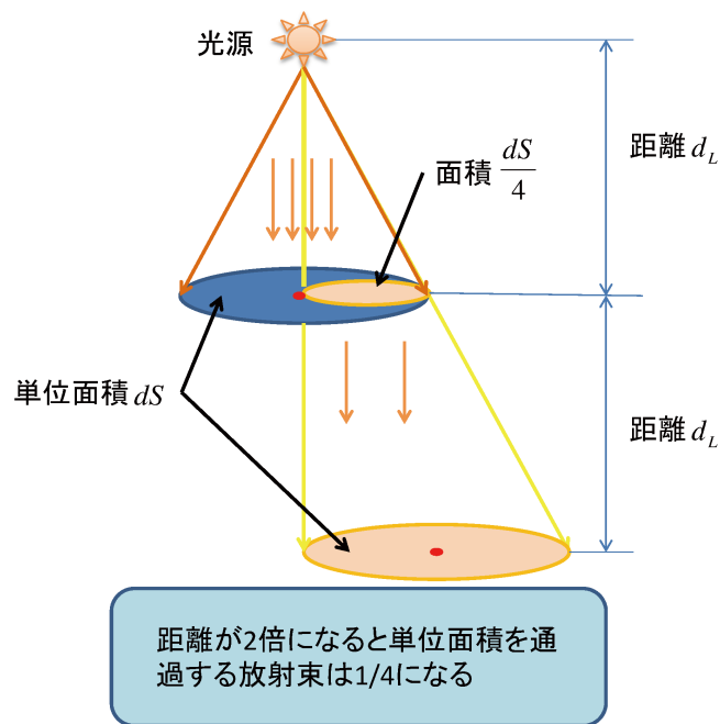
図 50 照度の逆二乗則
