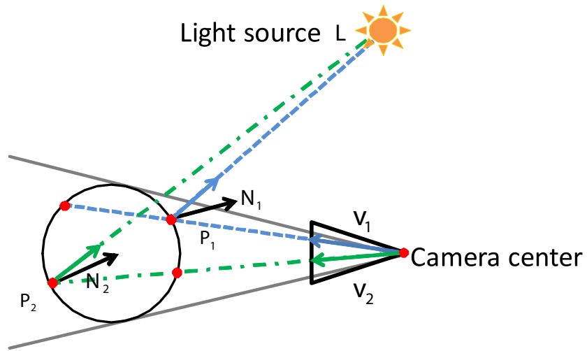
(a) 光源が透明球を含む視体積外に存在する場合
