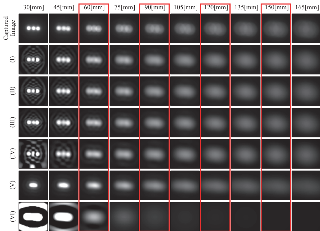
図 19 観測された画像および手法 (I)-(V) によって推定された放射輝度分布を用いてリライティングした画像. (I) L1 ノルム正則化と物理制約を用いた手法, (II) L1 ノルム正則化を用いた手法, (III) 物理制約を用いた手法, (IV) 制約を何も使わない手法, (V) 光源を非等方な放射輝度分布を持つ点光源であると仮定した手法, (VI) 光源を等方な放射輝度分布を持つ点光源の集合であると仮定した手法. 手法 (I)-(V) において実球面調和関数の次数を 34 とし放射輝度分布の推定を行った. 図中赤枠で囲まれた領域は放射輝度分布の推定に用いた撮影画像に対応している. なお図中の画像は拡大表示されている.
