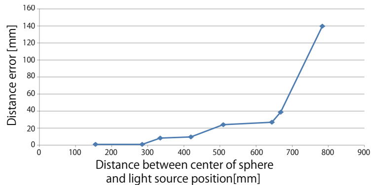
図 42 実環境における位置推定誤差
