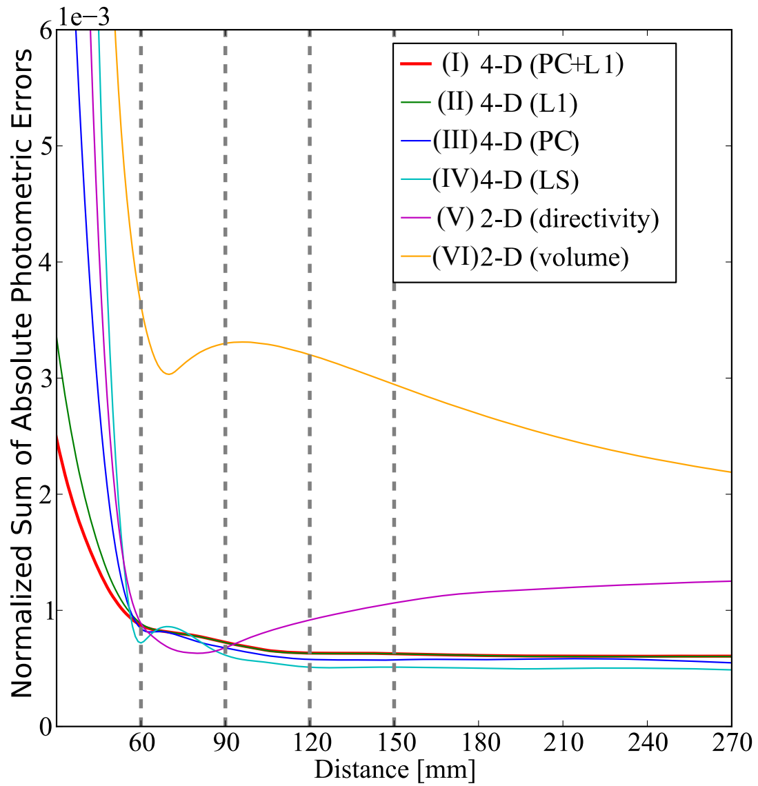
図 22 観測画像とリライティングした画像との輝度誤差. 図中灰色点線は入力画像が撮影された距離を示す.
