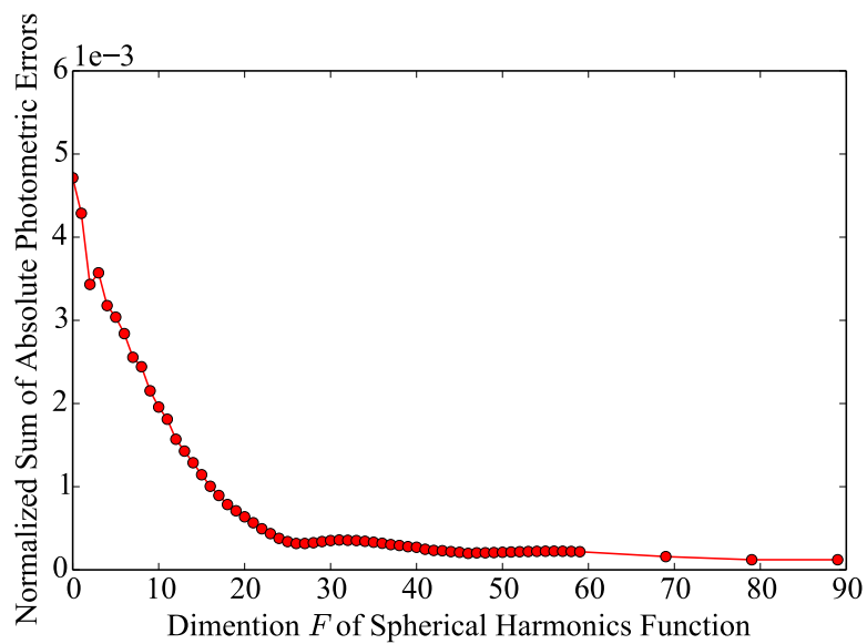
図 25 実球面調和関数の次数 F を変化させた場合における真値とリライティングした画像との輝度誤差
