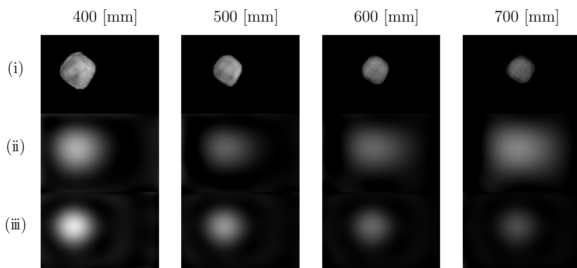
図 16 実環境において推定された放射輝度分布を用いてリライティングした画像. (i): 視体積制約を用いた手法. (ii) 制約を用いない手法. (iii) 光源を非等方な放射輝度を持つ点光源であると仮定した手法.
