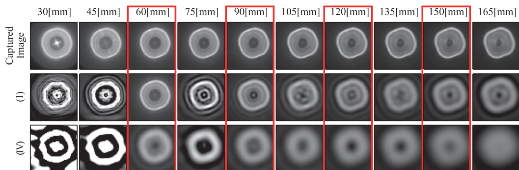
図 30 レンズとリフレクターが付随した光源を用いた場合における撮影画像 (真値) と各手法によって推定された放射輝度分布を用いてリライティングした画像. (I) L1 ノルム正則化と物理制約を用いた手法, (IV) 制約条件を用いない手法. 実球面調和関数の次元を 34 とし, 空間方向の解像度を 35 として放射輝度分布を推定. 図中赤枠で囲まれた領域は放射輝度分布の推定に用いた撮影画像に対応している. なお図中の画像は拡大表示されている.
