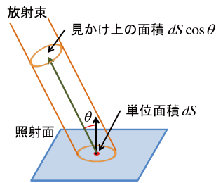
図 51 照度の入射角余弦則
