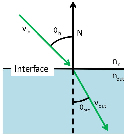
図 34 スネルの法則
