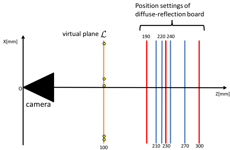
(a) カメラ・光源・ディフューザの位置関係. 図中黄色丸は光源位置を表し, 上から L-G-I-H-T の文字を投影する光源であり, 図中オレンジ線はライトフィールド平面 \mathcal{L} の設定位置を表す. また図中の青線は入力に用いた撮影画像のディフューザ設置位置を表し, 図中の赤線は入力に用いなかった撮影画像のディフューザ設置位置を表す.
