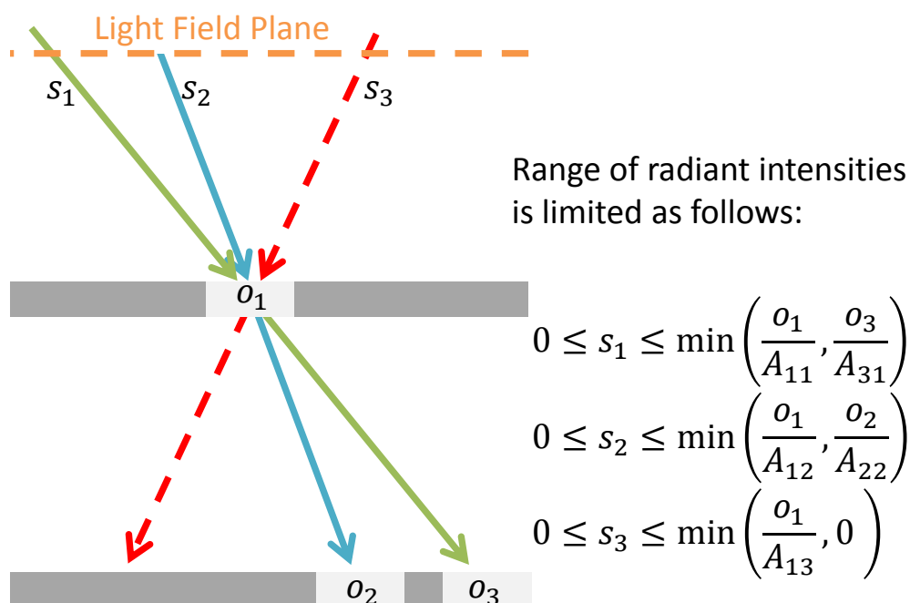
図 9 光線強度の取り得る値を範囲を制限する物理制約. 図中灰色領域は照明によって照らされていない領域を表す.
