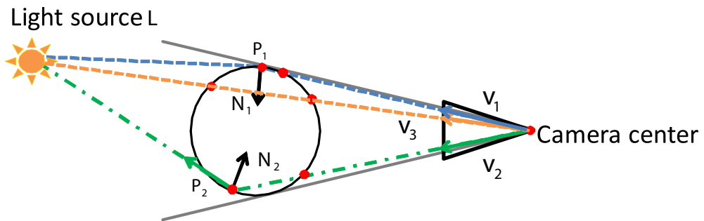
(b) 光源が透明球を含む視体積内に存在する場合
