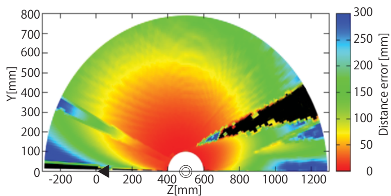
(a) 中空透明球体. 再投影誤差最小化 ( \sigma = 1.0 , 厚さ 2\text{mm} , 屈折率 1.5) 球の厚みを無視して光源位置を推定
