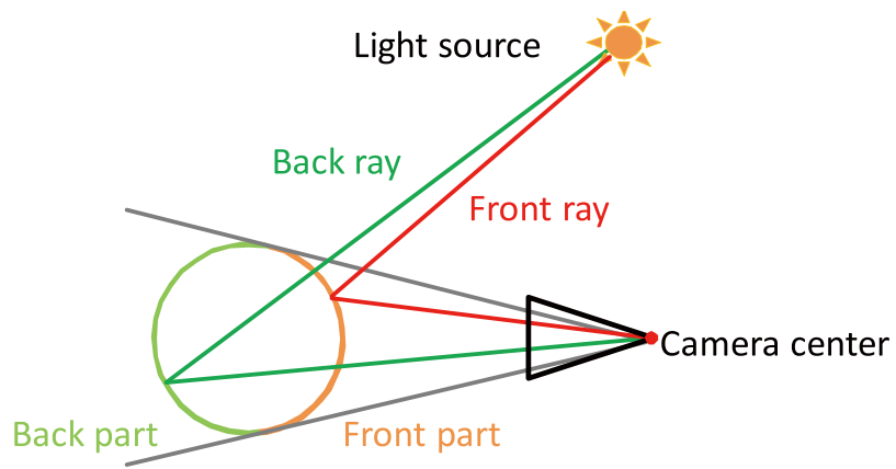
(a) 球面前部・後部反射光
