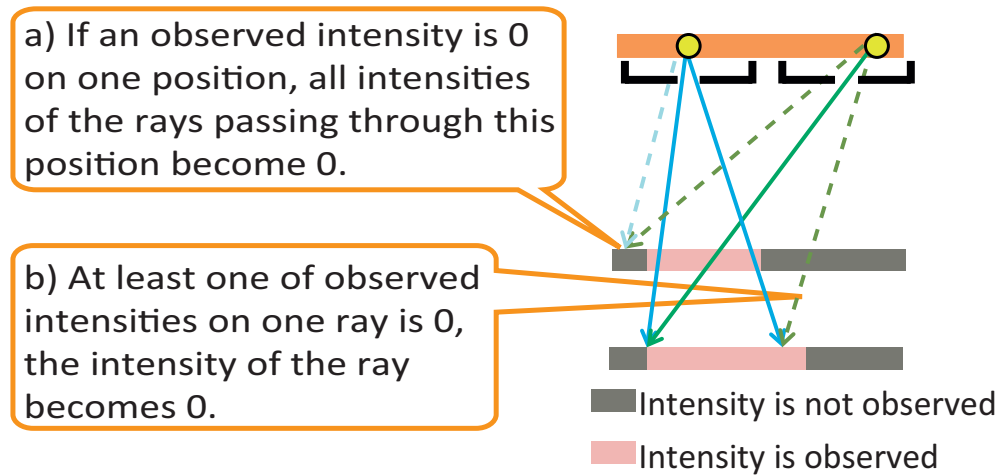
図 8 光線の視体積制約の外観図. 図中灰色領域は照明によって照らされていない領域を表し, 図中桃色領域は照明によって照らされている領域を表す.
