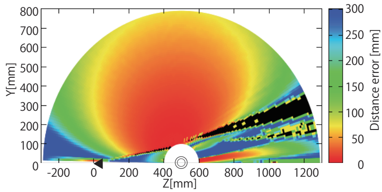
(a) 中空透明球体. 中点法 ( \sigma = 1.0 , 厚さ 0mm )
