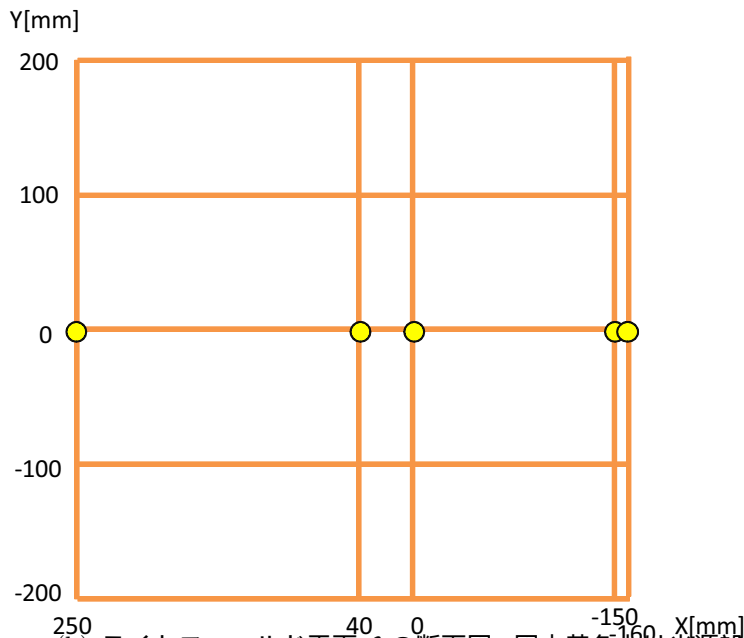
(b) ライトフィールド平面 \mathcal{L} の断面図. 図中黄色丸は光源設置位置を表し, 左から L-G-I-H-T の文字を投影する光源である. 図中の交点が放射輝度分布を推定した空間方向サンプリング位置を表す.
