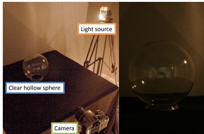
図 3 中空透明球体. 左: 実験環境の外観図 右: 観測画像
