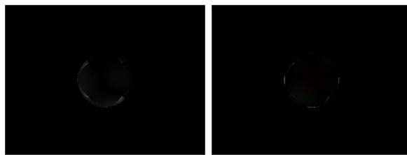
(d) 距離の差分画像 (e) 法線方向の差分画像
