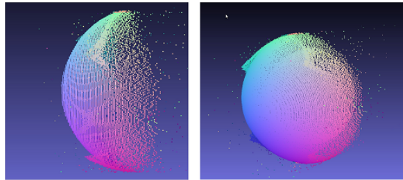
(b) 推定された光源位置情報を用いて復元された三次元点群
