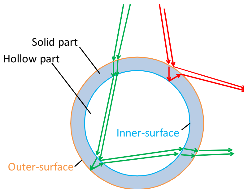
(b) 球面内部表面・外部表面反射光
