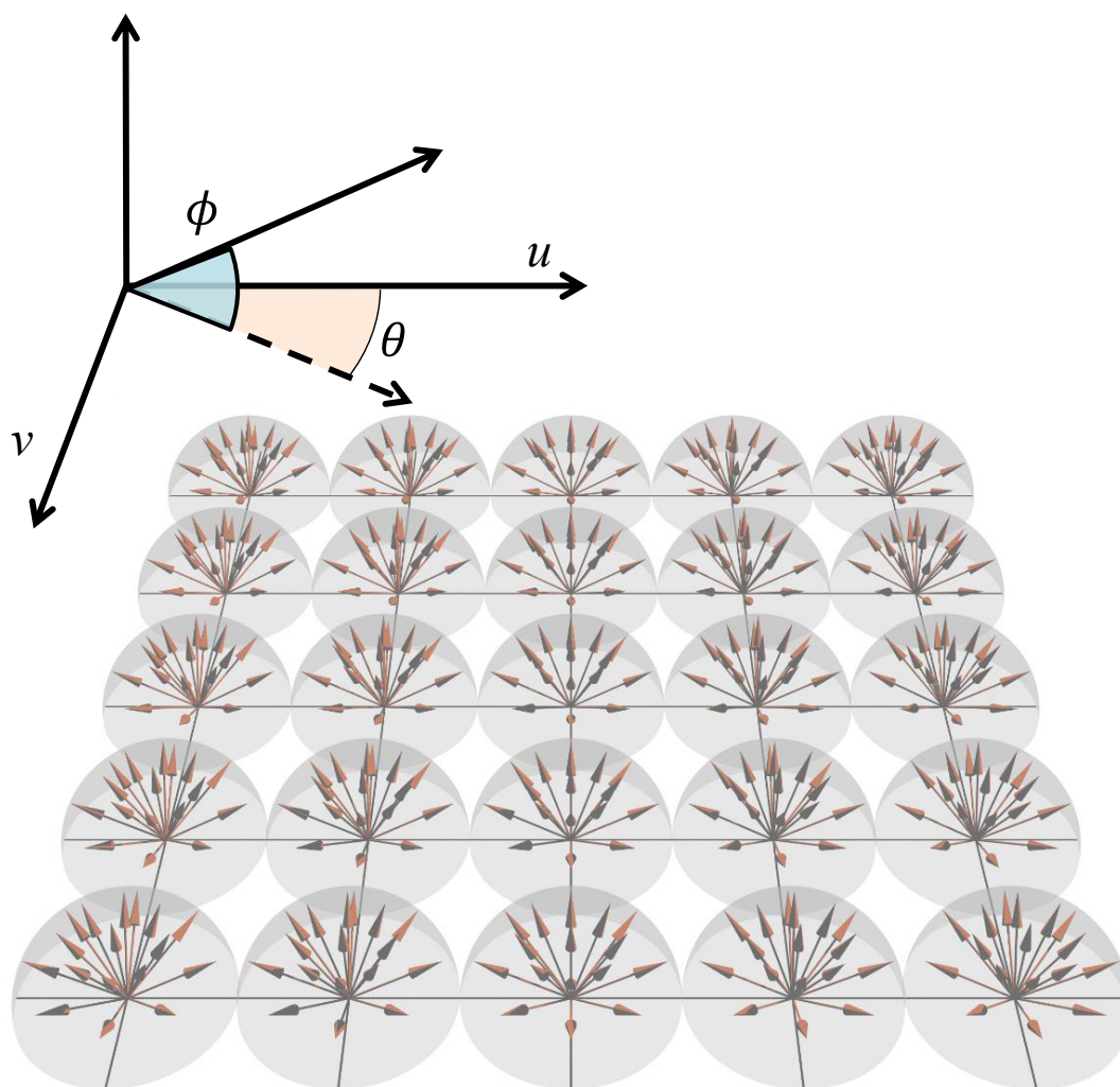
図 7 ライトフィールド平面 \mathcal{L} 上におけるライトフィールドのパラメータ化.
