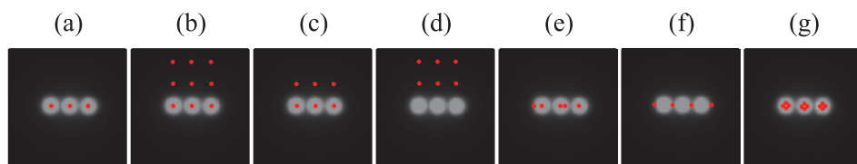
図 26 空間方向の分解能を変化させた場合において空間方向サンプリング点として与えた位置. (a) 各光源のハイライト領域重心をサンプリング位置として与えた場合, (b) 各光源のハイライト領域重心とハイライトが観測されなかった領域 6 点をサンプリング位置として与えた場合, (c) 各光源のハイライト領域重心とハイライトが観測されなかった領域 3 点をサンプリング位置として与えた場合, (d) ハイライトが観測されなかった領域 6 点をサンプリング位置として与えた場合, (e) 各光源のハイライト領域重心およびその周辺をサンプリング位置として与えた場合, (f) 各光源のハイライト領域重心を通過する直線上のハイライト領域と直線の交点の 4 点をサンプリング位置を与えた場合, (g) 各光源のハイライト領域重心位置の周辺の 4 点をサンプリング位置として与えた場合. 図中の赤丸は空間方向のサンプリング位置を表す. なお図中の画像は拡大表示されており, 図中灰色領域は距離 d = 0 において撮影を行った際における画像の明るさを半分にした画像である.
