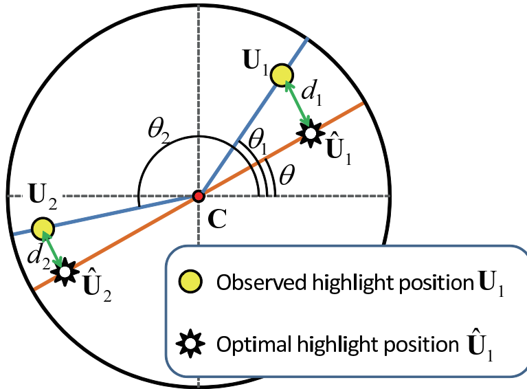
図 33 再投影誤差
