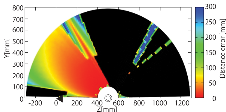
(a) 中実透明球体. 再投影誤差最小化 ( \sigma = 1.0 , 屈折率 1.5)
