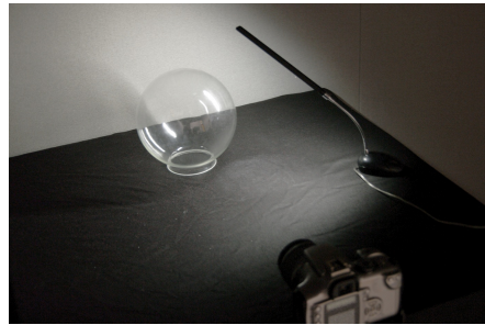
(b) 実験環境外観図
