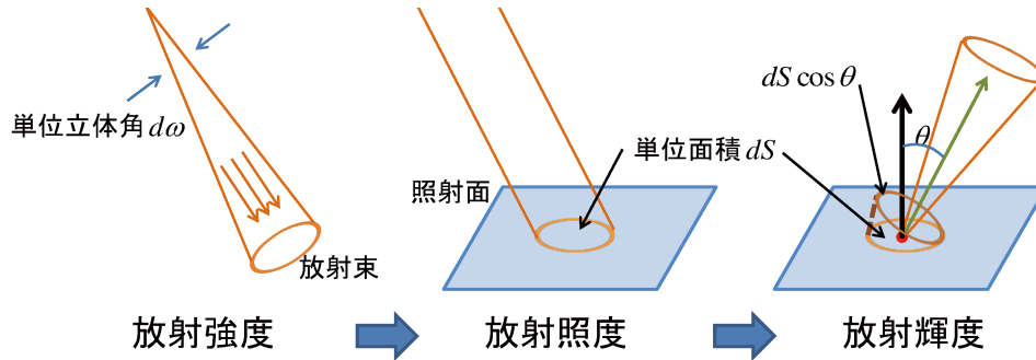
図 48 放射強度, 放射照度, 放射輝度
