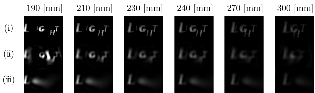
図 12 推定された放射輝度分布を用いてリライティングした画像. (i): 視体積制約を用いた手法. (ii) 制約を用いない手法. (iii) 光源を非等方な放射輝度分布を持つ点光源と仮定した手法.
