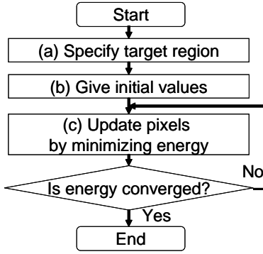
図 1 画像修復の処理の流れ Fig.1 Procedure of the proposed image inpainting method.
