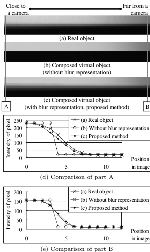
図 7 評価に用いた画像とエッジ部分での輝度変化の比較 Fig. 7 Images for evaluation and comparison of edge part of each image.
