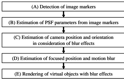
図 1 提案手法の処理の流れ Fig. 1 Flow diagram of the proposed method.
