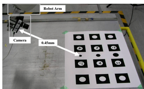
図 9 ロボットアームを用いた実験環境 Fig.9 Experimental environment with robot arm
