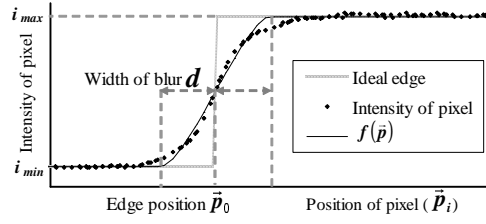
図 4 ぼけエッジに対する関数当てはめ
