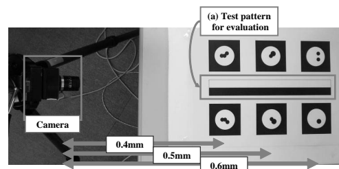
図 5 実験環境
